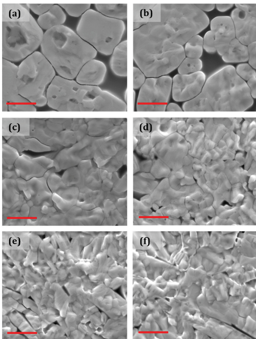
Figure 4. Scanning electron microscopy images of films annealed for periods of a) 60 min, b) 80 min, c) 100 min, d) 120 min, e) 140 min, and f) 180 min. Red scale bars correspond to 1 \mu\text{m} .
